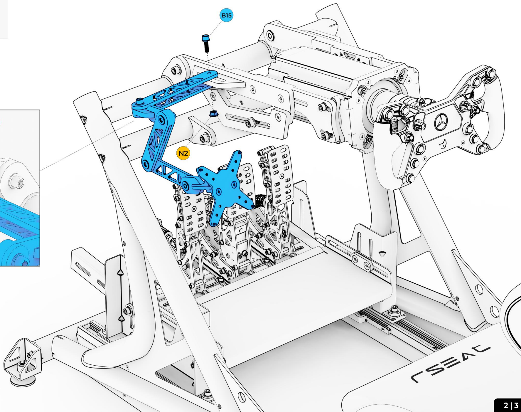
N2 M8 NUT DIN 6923
