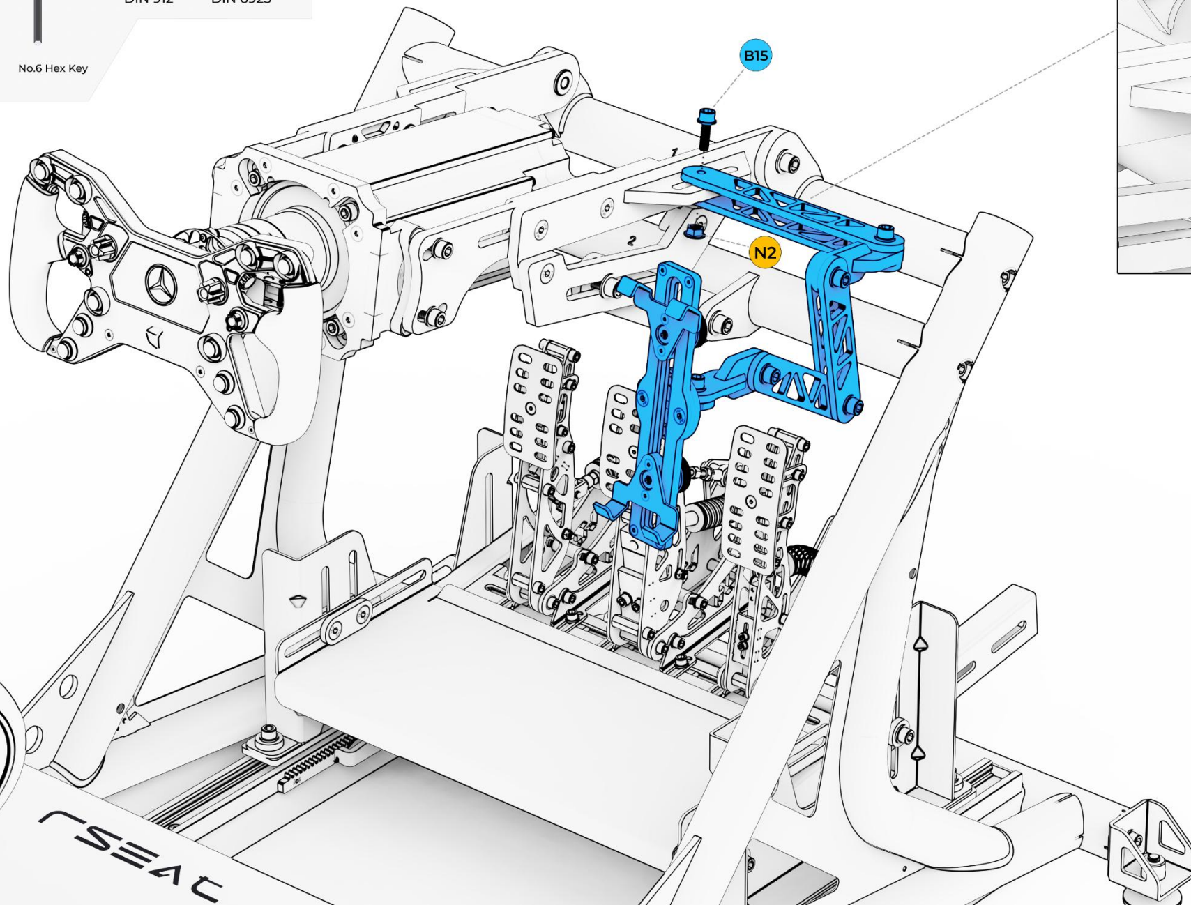
B15 M8x25 DIN 912
