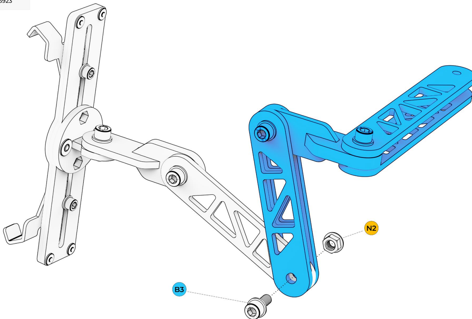
N2 M8 NUT DIN 6923
